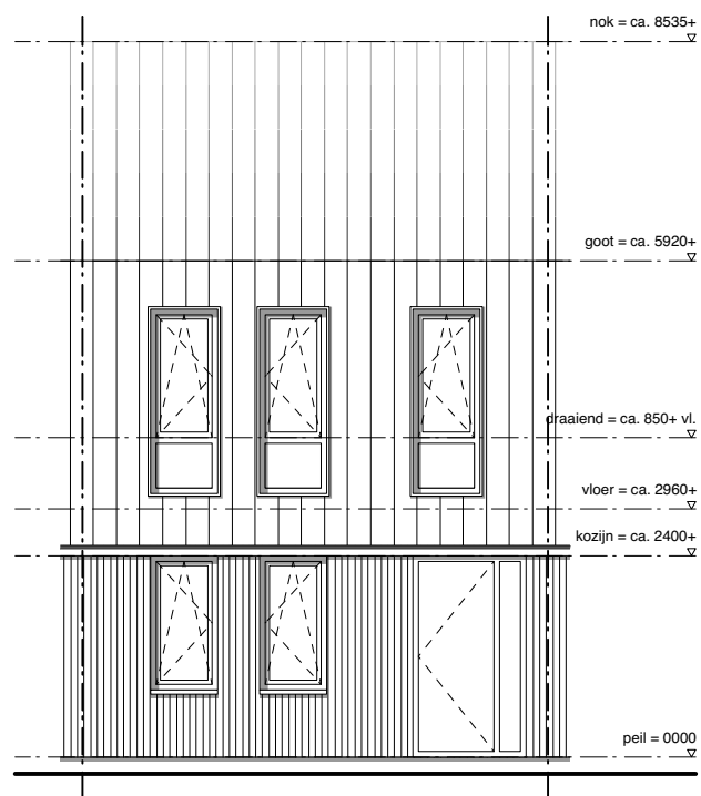
VOORGEVEL
