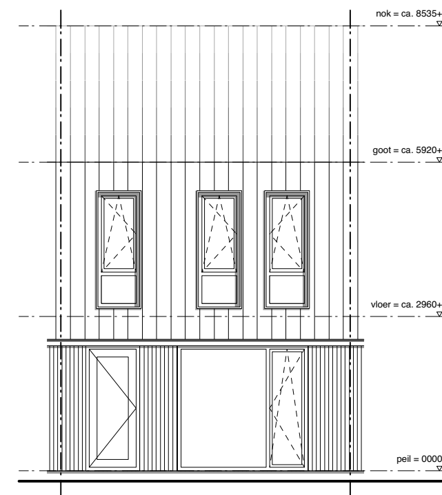
ACHTERGEVEL
